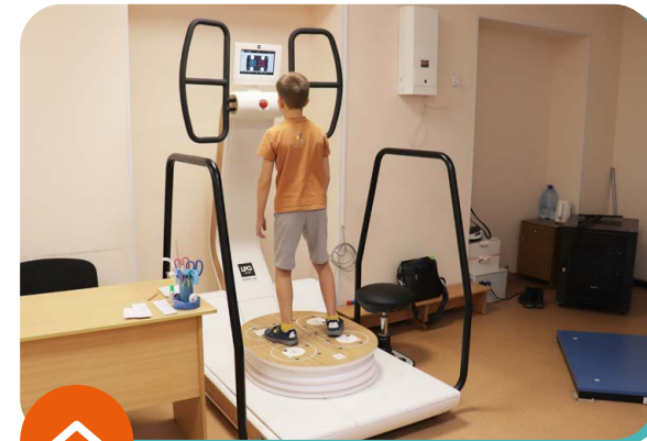
Система нейромышечной реабилитации и диагностики с БОС
